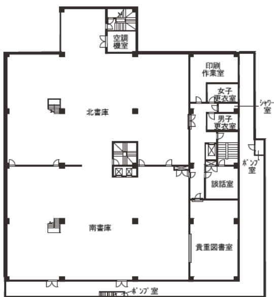
地下2 階
