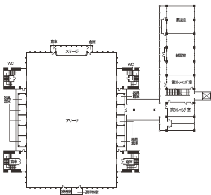
2 階
